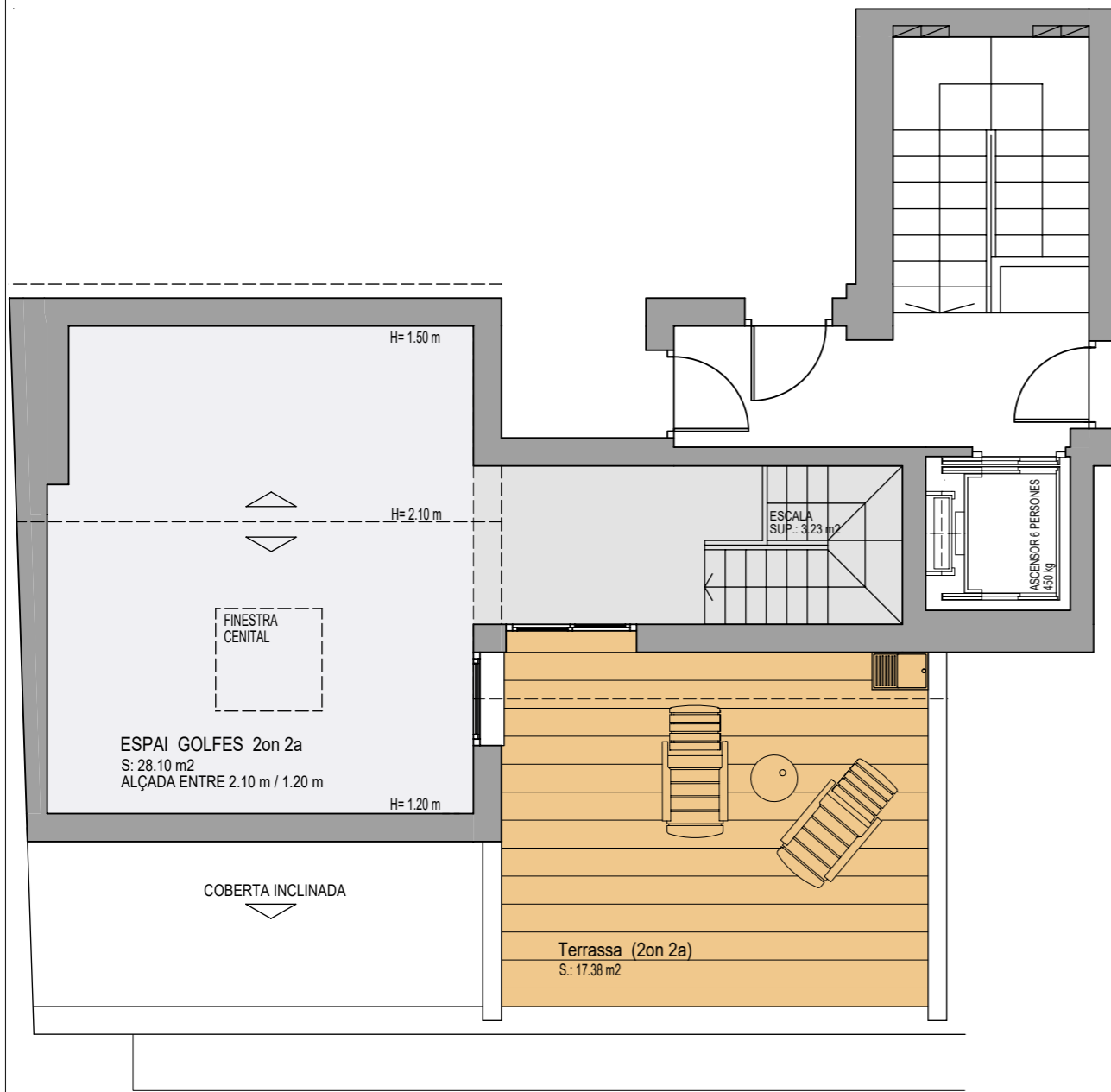
PLANTA SOTACOBERTA
