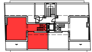
PLANTA SOTACOBERTA
